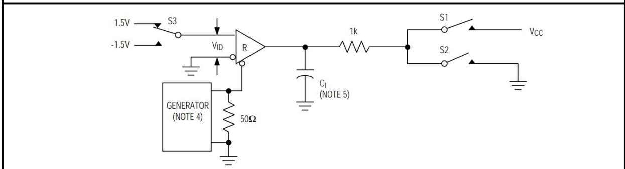
图 7 接收器传播延时测试电路
